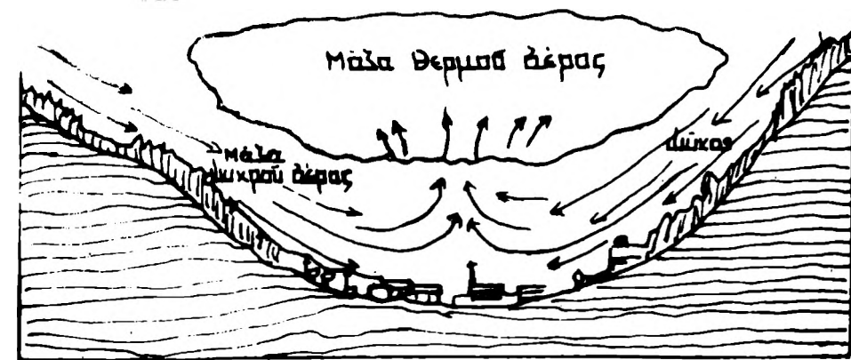
Θερμοκρασιακή αναστροφή
